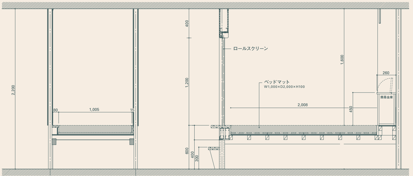
【正面図】
